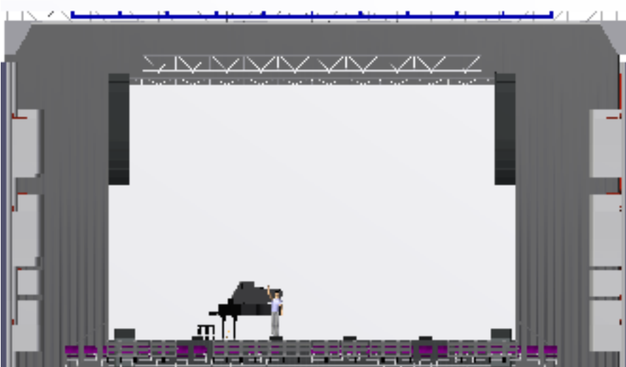
2 Arena Front Scale: 1/16" = 1'-0"
